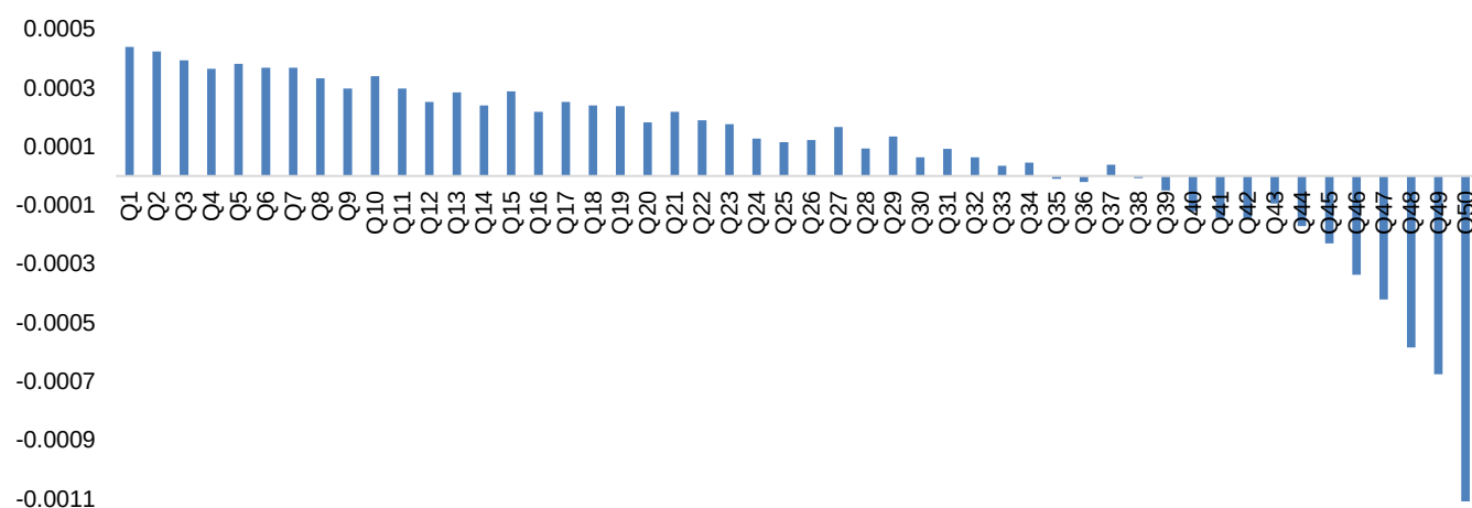
图 7: BuyTransaction_BuyOrder_ratio_09150925因子在深证A指成分股中的50档分档表现
